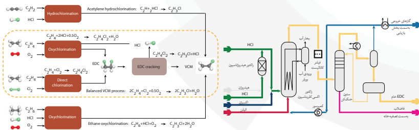
شکل ۳- تولید VCM از طریق سه روش: هیدروکلریناسیون استیلن، کلریناسیون/هیدروکلریناسیون مستقیم اتیلن و اکسی کلریناسیون اتان [۶].
